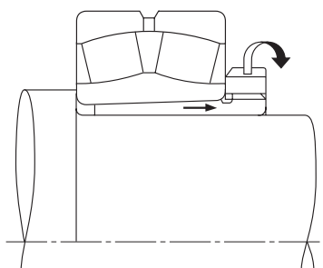
Рис.14.16. Удаление стяжной втулки с помощью отводной гайки (1)
