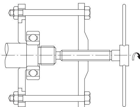
Рис. 14.13. Демонтаж внутреннего кольца с помощью съемника (1)
