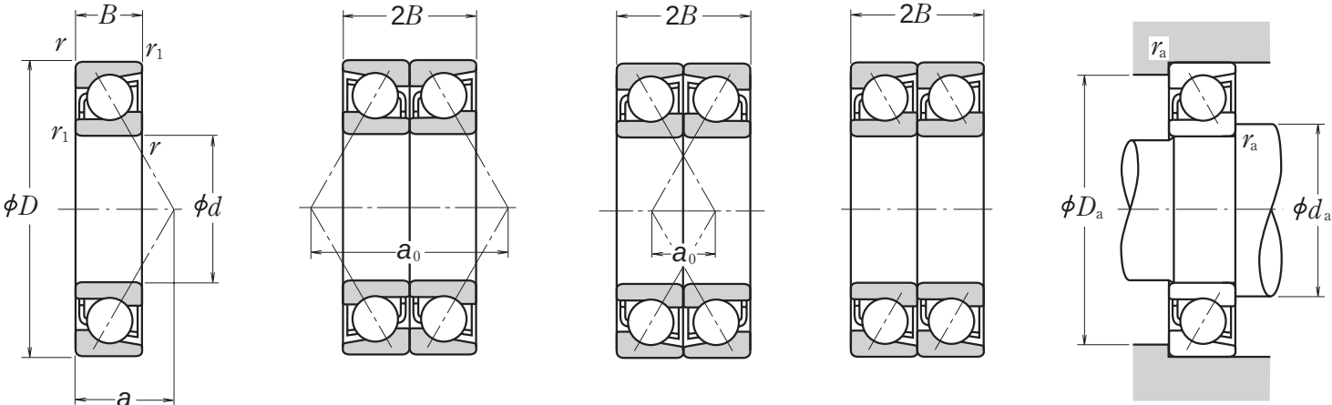
Одиночный По О-образной схеме DB По Х-образной схеме DF По схеме Тандем DT
