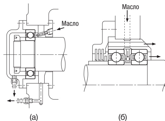
Рис. 12.8. Смазка впрыскиванием
