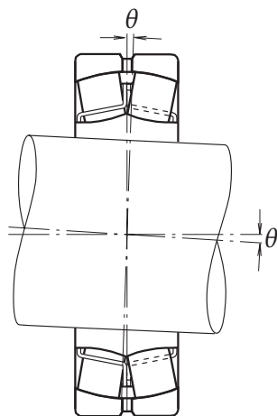
Рисунок 3.4. Допустимая несоосность сферических роликоподшипников
