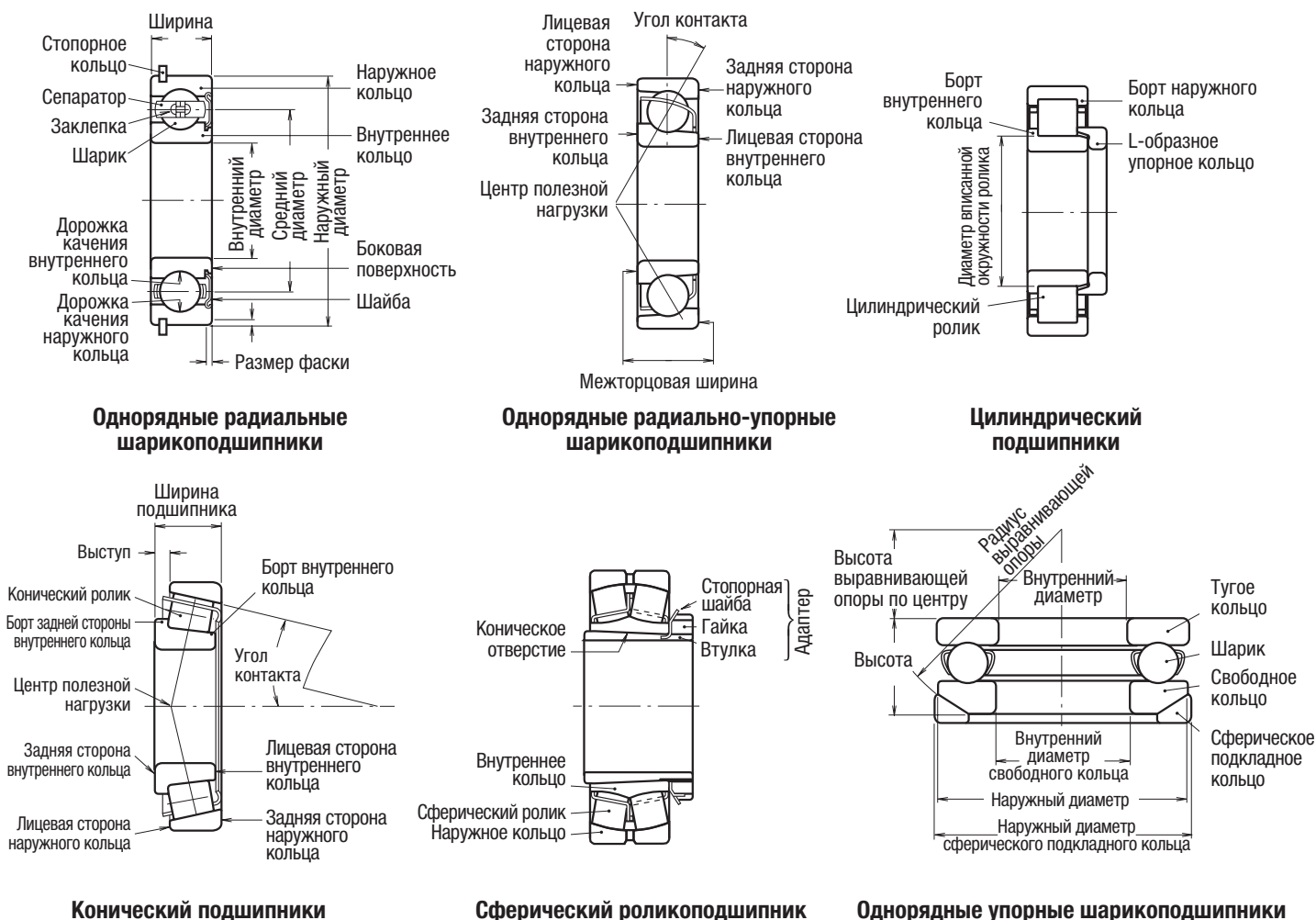
Рисунок 1.1 Терминология подшипниковых деталей
