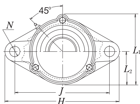
Тип с литой пылезащитной крышкой
