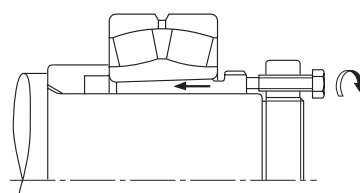
Рис. 14.5. Посадка подшипника со стяжной втулкой
