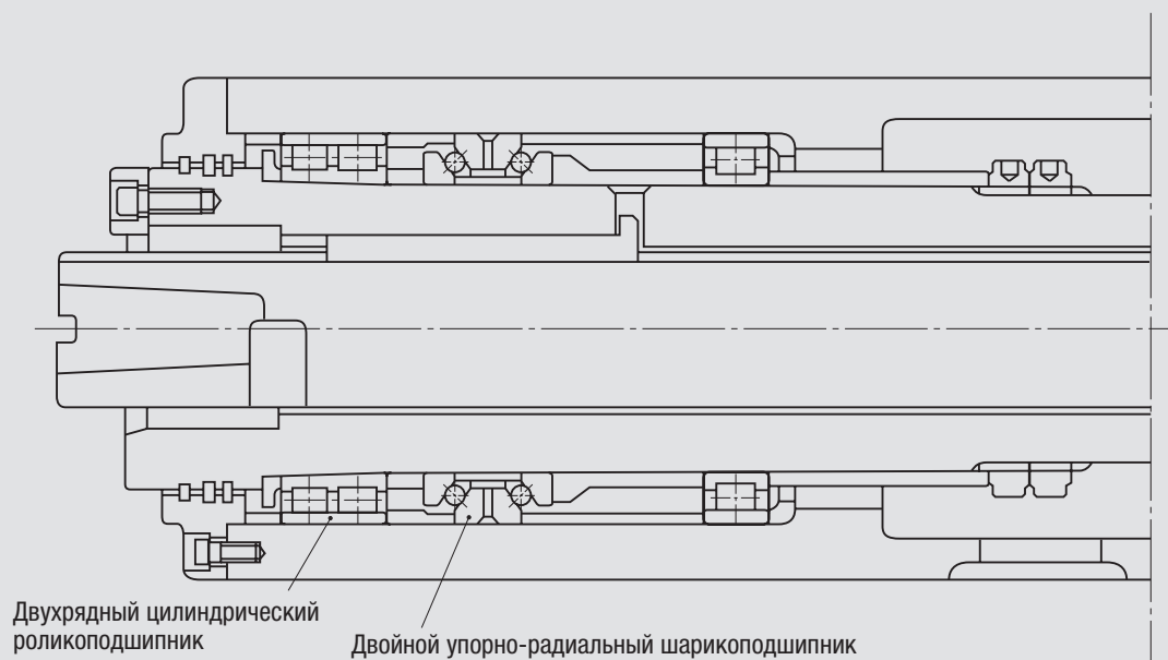
Пример применения двойного упорно-радиального шарикоподшипника (главный шпиндель обрабатывающего станка)
