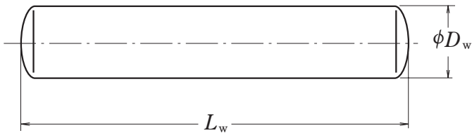
Ролик со сферической торцевой поверхностью
