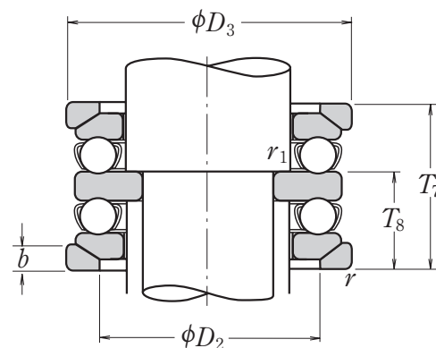
Со сферическим подкладным кольцом
