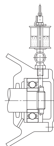
Рис. 12.5. Капельное смазывание
