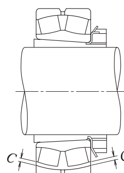
Рис. 14.8. Измерение зазора в сферическом роликоподшипнике
