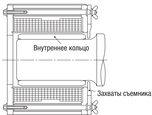
Рис. 14.15. Демонтаж внутреннего кольца с помощью индукционного нагревателя
