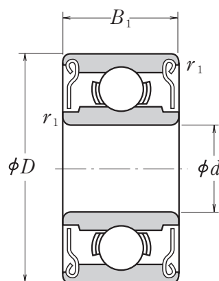
Тип с защитными шайбами ZZ · ZZ1
