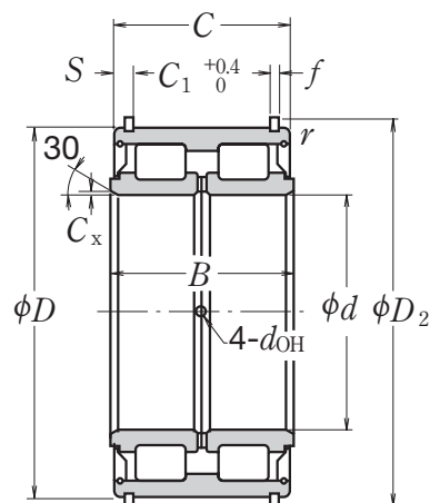
С установочным кольцом
