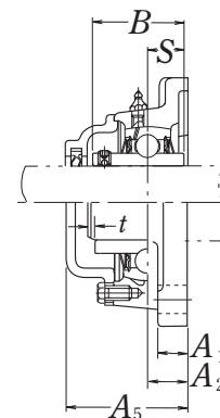
Тип с литой пылезащитной крышкой
