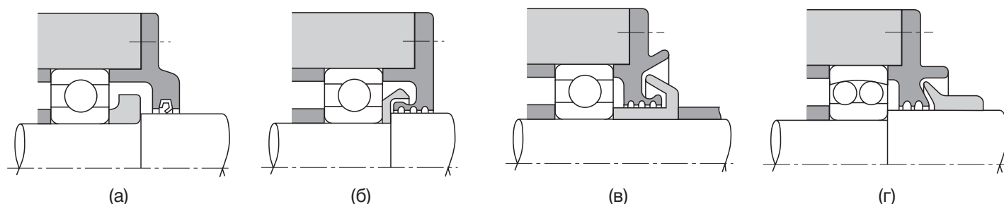
Рис. 11.6. Примеры конфигураций маслоотражательных колец
