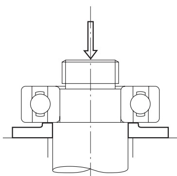
Рис. 14.12. Демонтаж внутреннего кольца с помощью пресса
