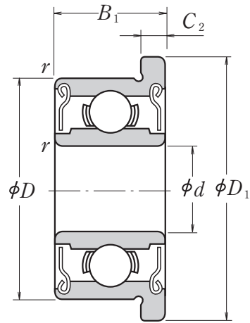
Тип с защитными шайбами ZZ · ZS
