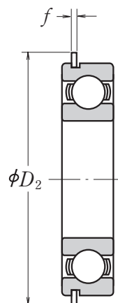
Со стопорным кольцом NR
