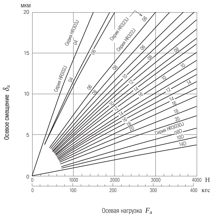
Рис. 15.4. Осевая нагрузка и осевое смещение конических роликоподшипников
