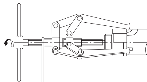
Рис.14.14. Демонтаж внутреннего кольца с помощью съемника (2)
