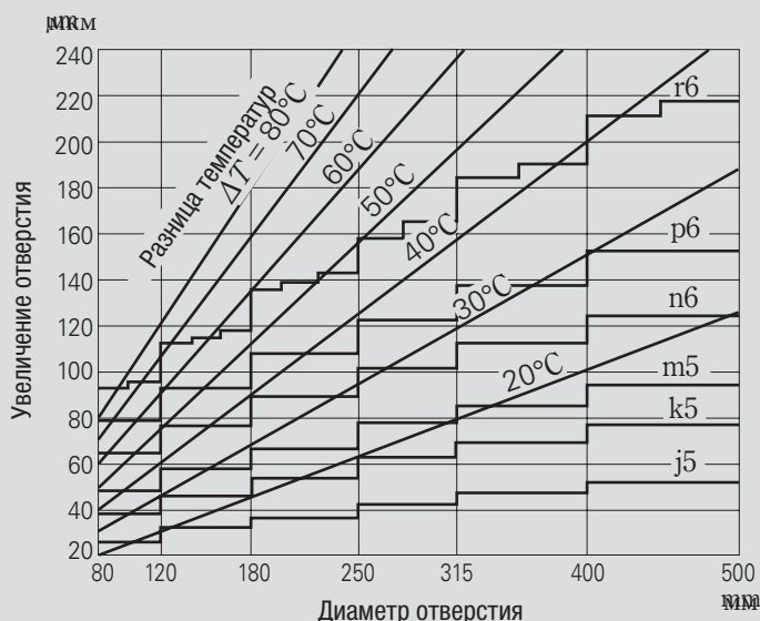
Рис. 14.3. Температура и тепловое расширение внутреннего кольца
