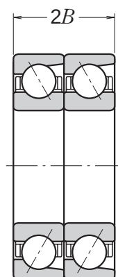
По схеме Тандем DT
