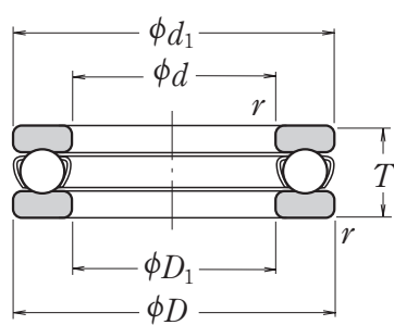
С плоской опорной поверхностью
