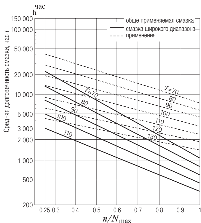
Рис. 12.3. Долговечность смазки в закрытых шарикоподшипниках
