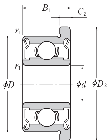
Тип с защитными шайбами ZZ · ZZ1
