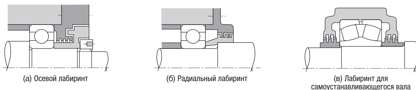
Рис. 11.7. Примеры конструкций лабиринтных уплотнений
