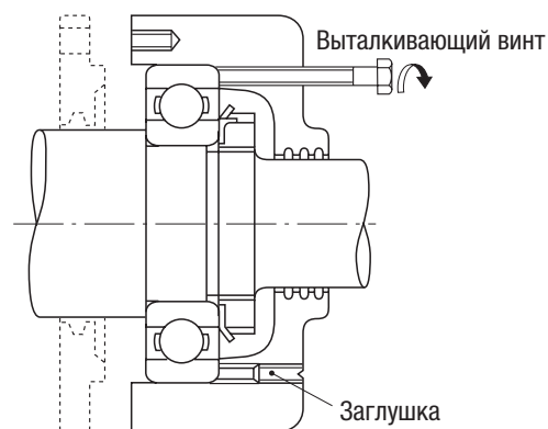
Рис.14.10. Демонтаж наружного кольца при применении выталкивающих винтов
