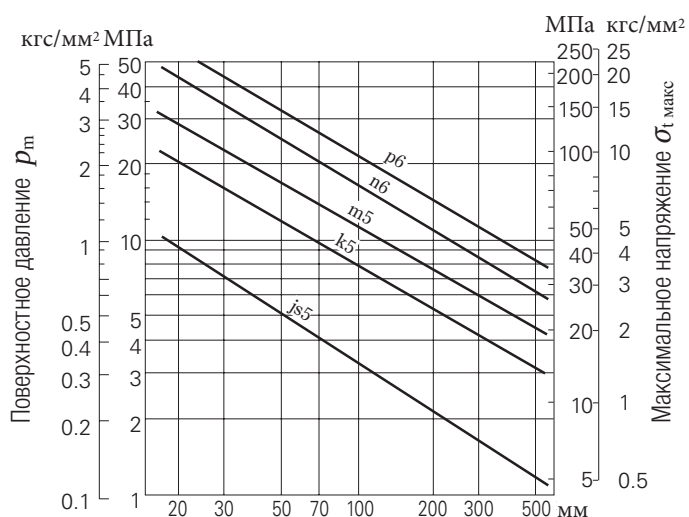
Рис.15.5. Поверхностное давление p_m , а также максимальное напряжение \sigma_{t \text{ макс}} для среднего натяга
