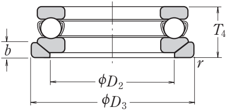
Со сферическим подкладным кольцом
