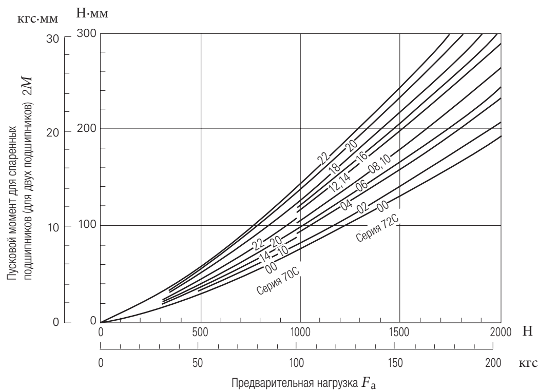
Рис. 15.11. Предварительная нагрузка и пусковой момент для радиально-упорных шарикоподшипников, установленных по схеме «Х» и «О» ( \alpha = 15^\circ )
