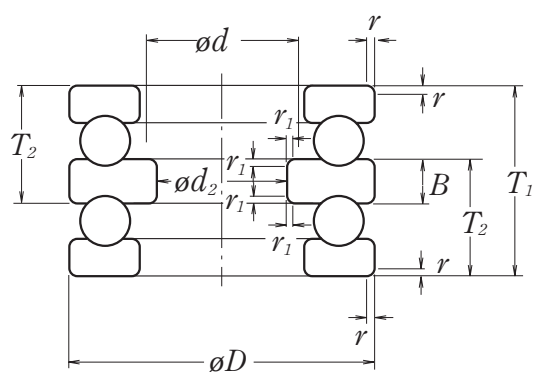
Рис. 7.4. Двойные упорные шарикоподшипники
