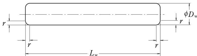
Ролик с плоской торцевой поверхностью
