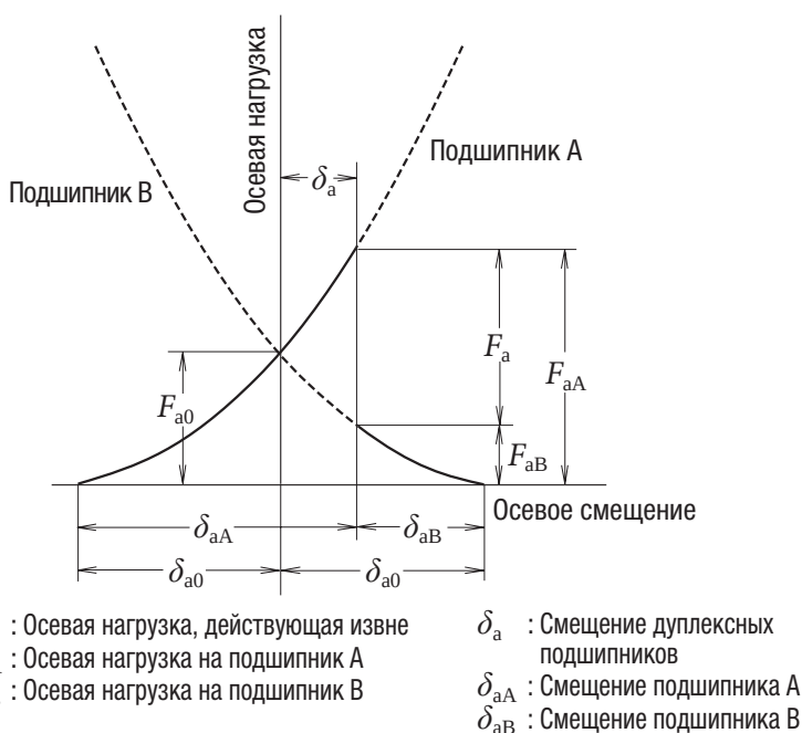
Рис. 10.4. Осьевое смещение при создании предварительного натяга при установке
