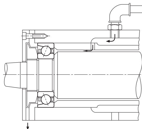
Рис. 12.9. Смазка масляным туманом
