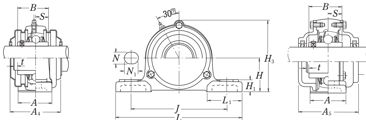
Тип с литой пылезащитной крышкой
