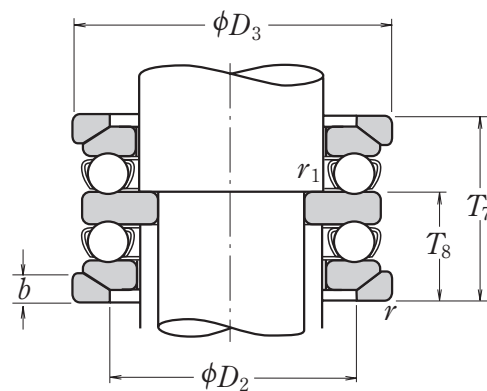
Со сферическим подкладным кольцом
