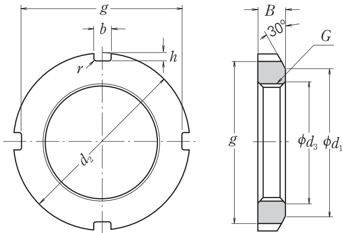
Гайка с шайбой
