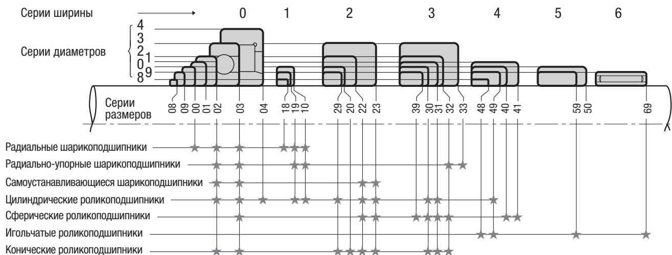
Рисунок 3.1. Размерные серии радиальных подшипников
