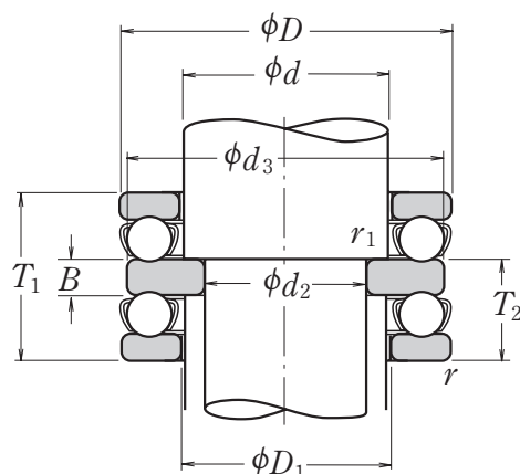
С плоской опорной поверхностью
