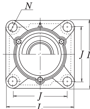
Тип с литой пылезащитной крышкой
