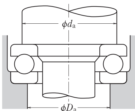
Рис. 11.3. Диаметры опорной поверхности для упорных шарикоподшипников
