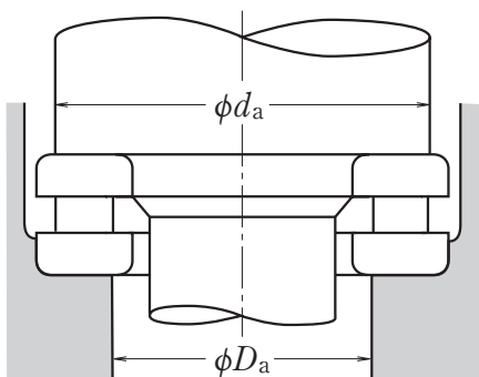
Рис. 11.4. Диаметры опорной поверхности для упорных роликоподшипников
