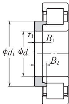
L-образные упорные кольца
