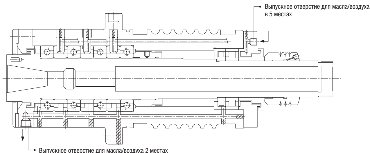
Рис.12.10. Масляно-воздушный метод смазки
