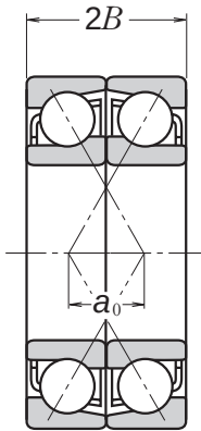
По X-образной схеме DF
