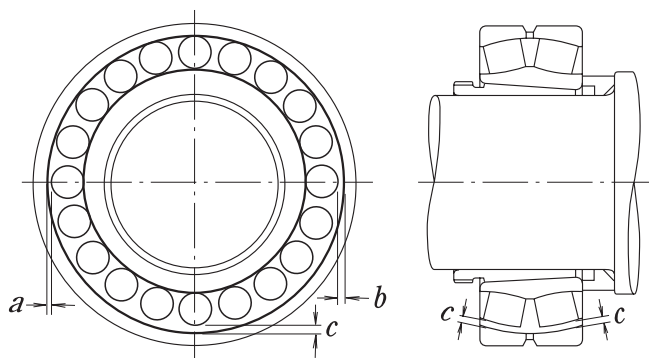
Рис. 14.9. Измерение зазора в крупногабаритных сферических роликоподшипниках
