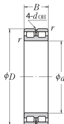
Подшипник свободного конца вала
