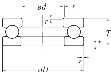
Рис. 7.3. Одинарные упорные шарикоподшипники
