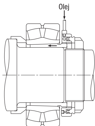
Рис. 14.6. Монтаж подшипника при помощи гидравлической гайки
