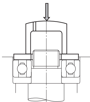
Рис. 14.2. Одновременная запрессовка внутреннего и наружного колец
