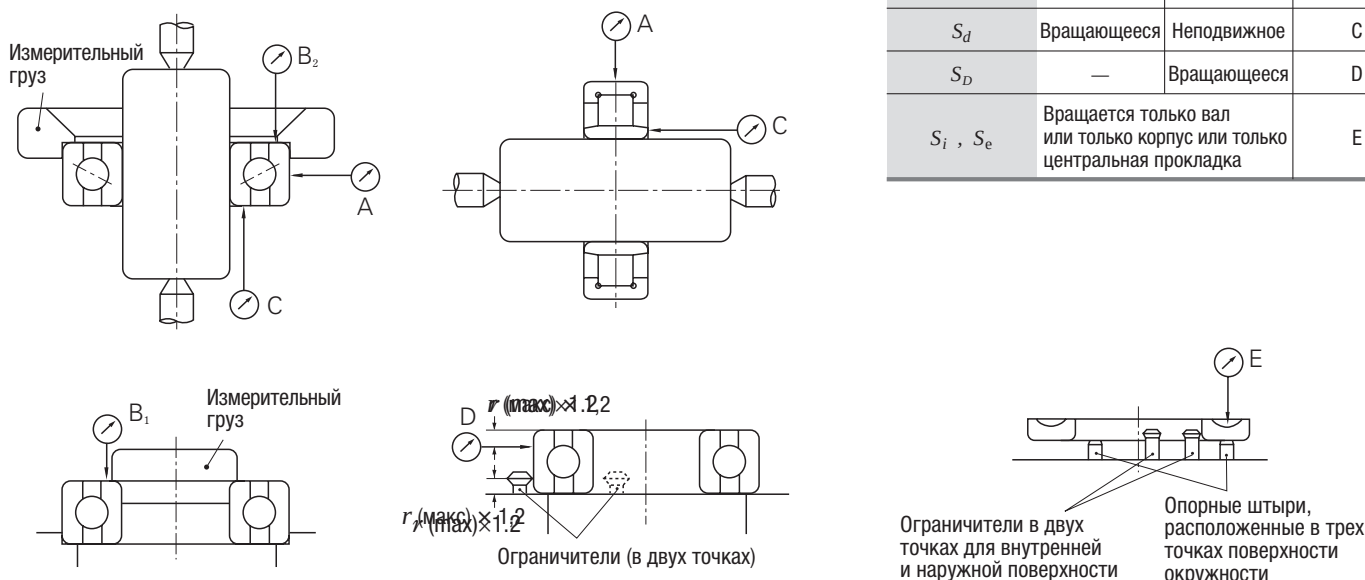
Рис. 8.1. Методы измерения точности вращения (обобщение)
