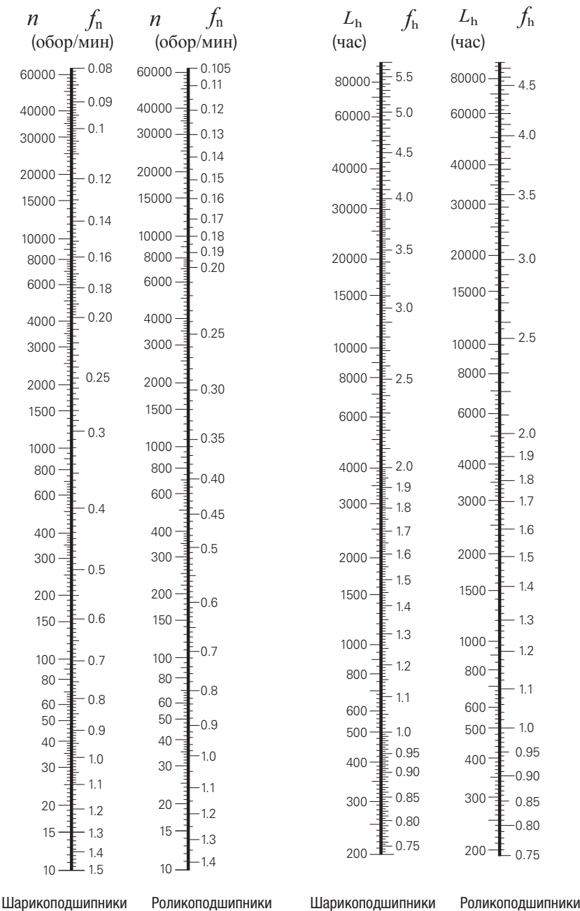
Рисунок 5.3. Скорость вращения подшипника и коэффициент скорости вращения
