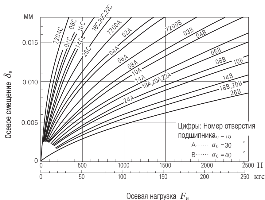
Рис. 15.3. Осевая нагрузка и осевое смещение радиально-упорных шарикоподшипников
