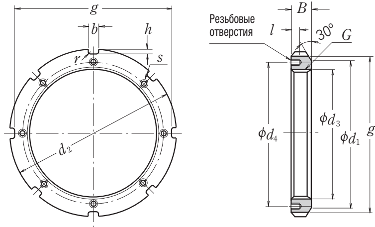
Гайка и фиксирующее устройство
