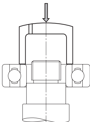
Рис. 14.1. Посадка внутреннего кольца с помощью пресса
