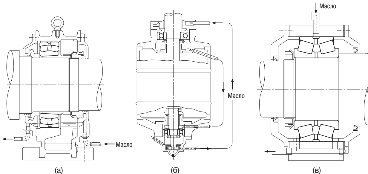
Рис. 12.7. Циркуляционная смазка
