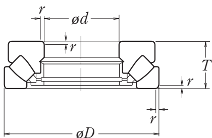
Рис. 7.5. Сферические упорные роликоподшипники
