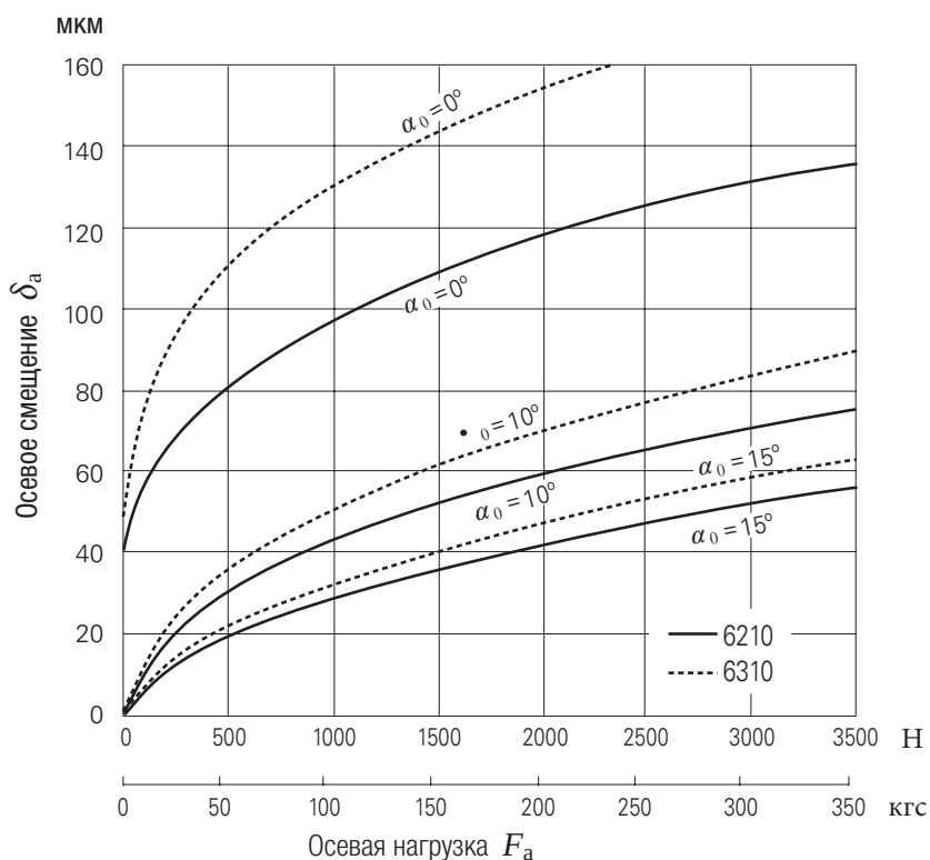
Рис. 15.2. Осевая нагрузка и осевое смещение радиальных шарикоподшипников
