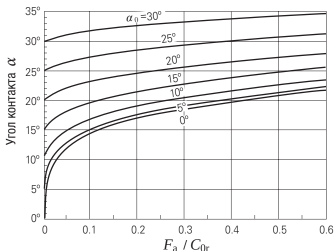
Рис. 15.1. F_a / C_{0r} и угол контакта радиальных и радиально-упорных шарикоподшипников
