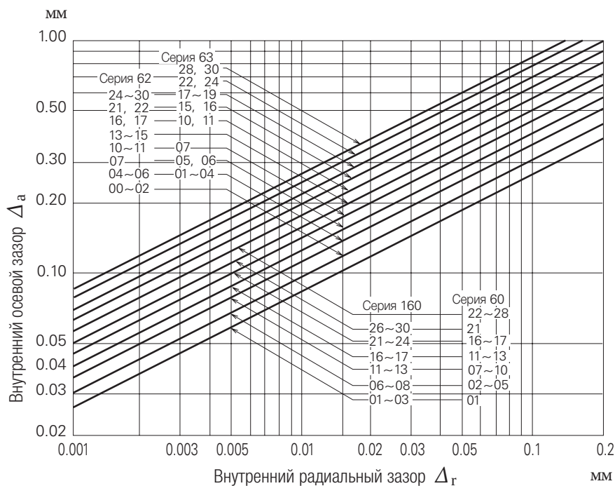
Рис. 15.7. \Delta_r и \Delta_a в однорядных радиальных шарикоподшипниках
