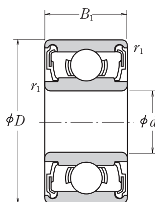
С контактным уплотнением DD
