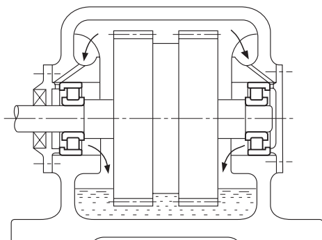
Рис. 12.6. Смазка разбрызгиванием
