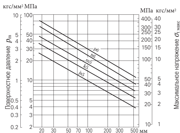
Рис.15.6. Поверхностное давление p_m , а также максимальное напряжение \sigma_{t \text{ макс}} для максимального натяга
