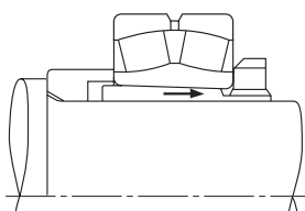
Рис. 14.4. Монтаж с закрепительной втулкой
