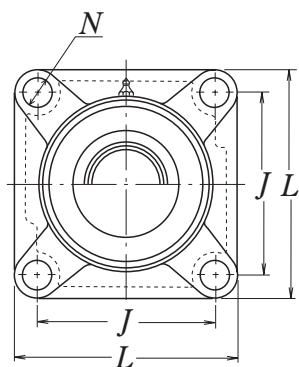
Тип со стальной штампованной пылезащитной крышкой
