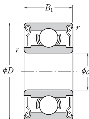
Тип с защитными шайбами ZZ · ZS
