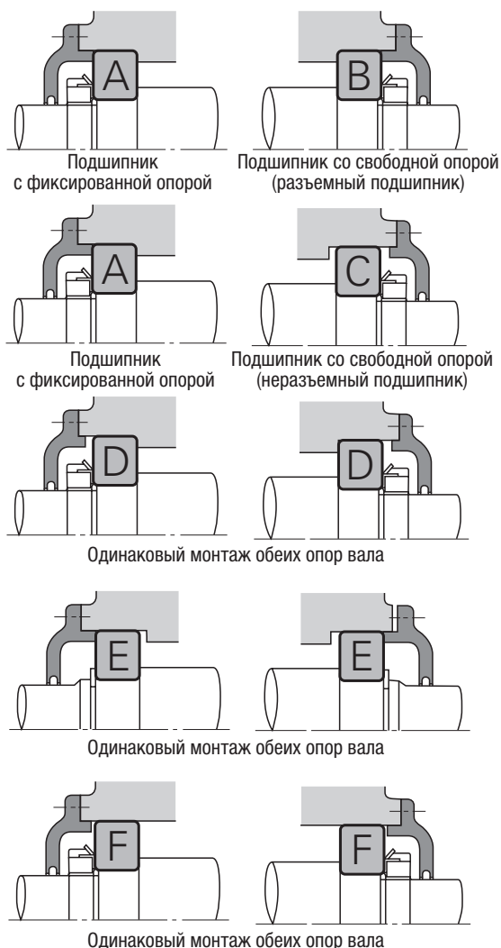
Рисунок 4.1. Выбор типа подшипника и способы монтажа
