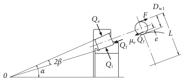
Рис. 15.9. Соотношение между e и \beta
