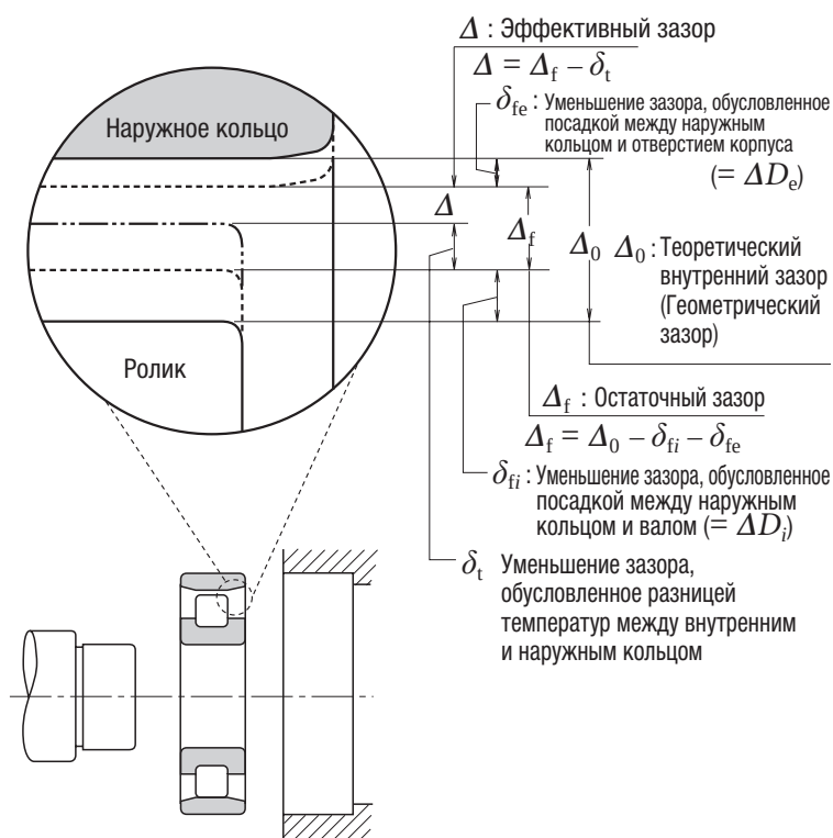
Рис. 9.2. Изменения внутреннего радиального зазора подшипников
