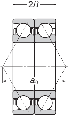
По O-образной схеме DB
