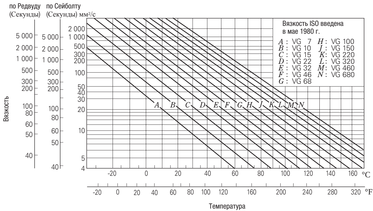
Рис. 12.11. Диаграмма температура – вязкость
