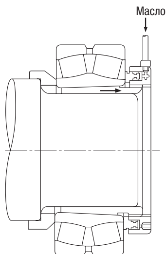
Рис.14.20. Демонтаж с помощью гидрогайки
