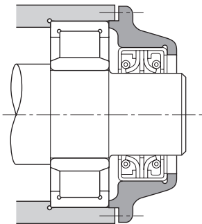
Рис.11.9. Пример применения масляного уплотнения (2)
