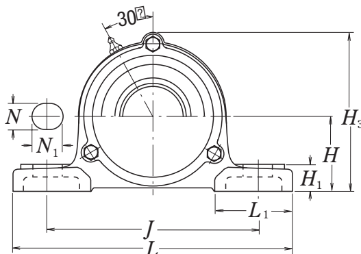
Тип с литой пылезащитной крышкой
