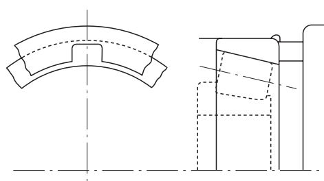
Рис.14.11. Канавки в корпусе конического роликоподшипника для демонтажа
