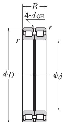
Подшипник фиксированного конца вала
