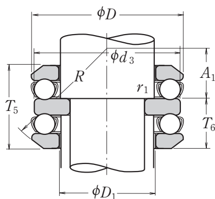
Со сферической опорной поверхностью
