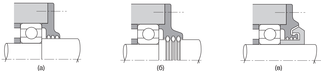
Рис. 11.5. Примеры смазочных канавок
