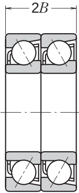
По схеме Тандем DT
