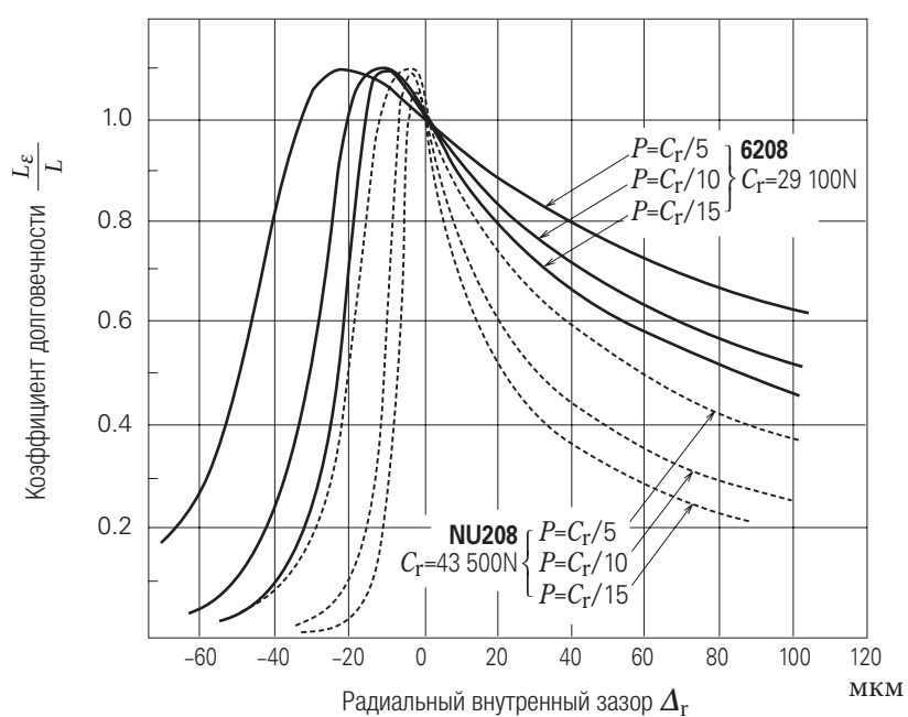
Рис. 15.13. Радиальный внутренний зазор и коэффициент долговечности
