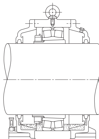
Рис. 12.4. Смазывание в масляной ванне
