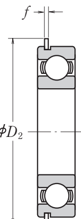
Со стопорным кольцом NR
