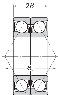
По 0-образной схеме DB
