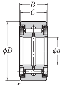
Без сепаратора, с уплотнением, с упорным кольцом
