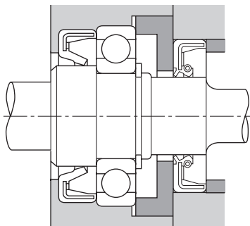
Рис. 11.8. Пример применения масляного уплотнения (1)
