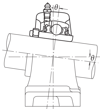
Рисунок 3.5. Допустимая несоосность шарикоподшипниковых узлов
