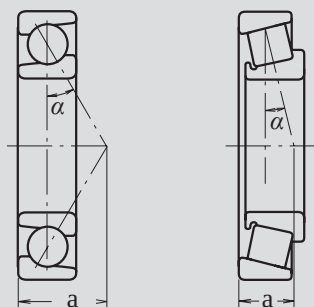
Рисунок 5.11. Центры эффективной нагрузки
