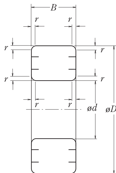
Рис. 7.1. Габаритные размеры радиальных шарикоподшипников и роликоподшипников
