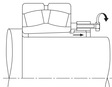
Рис.14.17. Удаление стяжной втулки с помощью отводной гайки (2)
