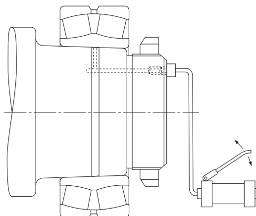
Рис.14.19. Демонтаж с помощью гидронасоса впрыскивающего масло
