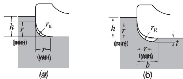
Рис. 11.2. Размеры фасок, радиуса галтели и высоты запле­чиков
