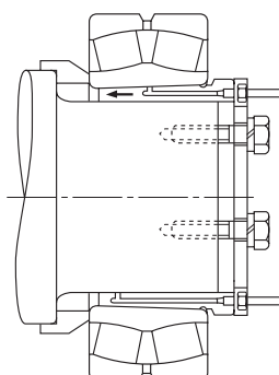
Рис. 14.7. Посадка подшипников со специальной втулкой и гидропрессом
