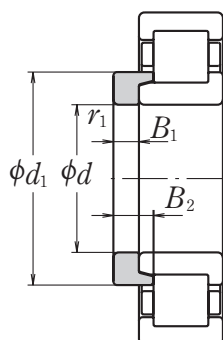
L-образные упорные кольца
