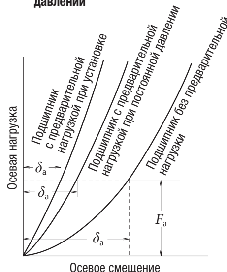
Рис. 10.6. Сравнение жесткости и методов предварительной нагрузки
