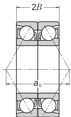
По O-образной схеме DB
