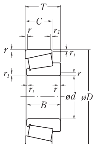
Рис. 7.2. Конические роликоподшипники
